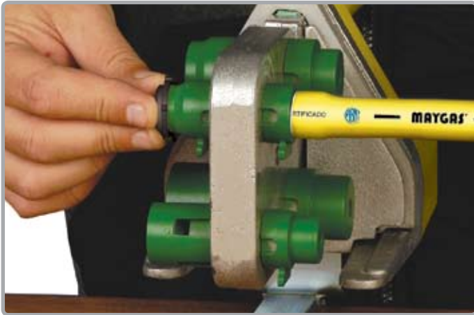
Primera termofusión
