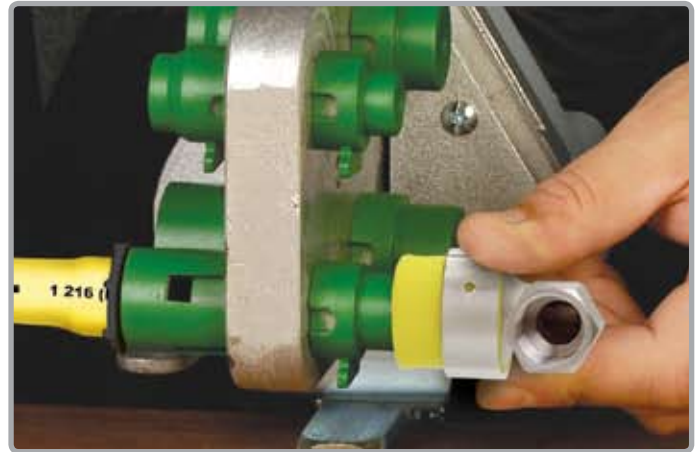
Segunda termofusión
